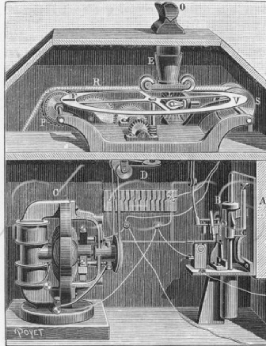
Fig. 5. — Mécanisme moteur du Kinétoscope.
